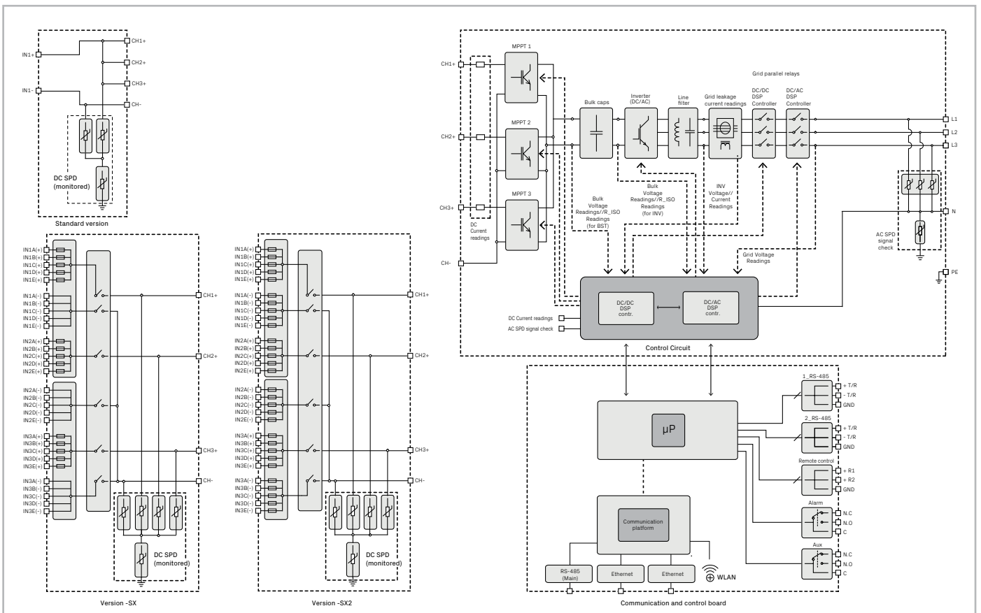
PVS-50/60-TL-String-Wechselrichter-Blockdiagramm
